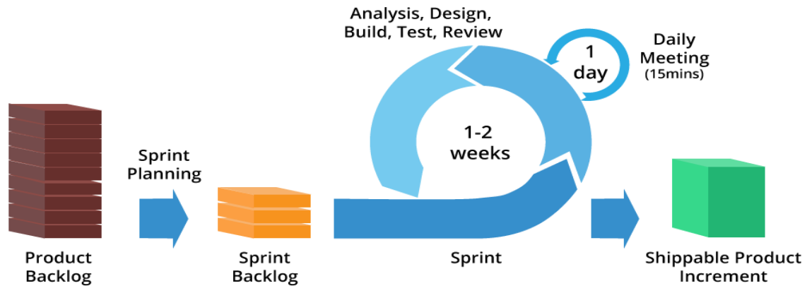
Figura. 1.4. Ciclo de vida del Sprint
