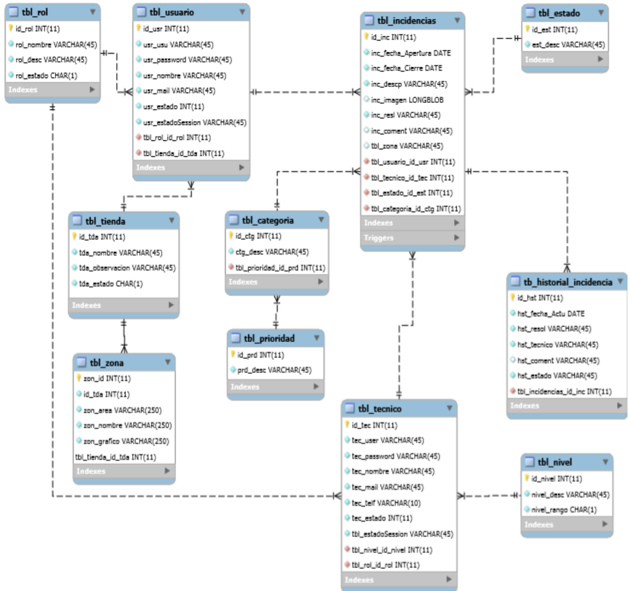
Figura. 4.1. Diagrama Entidad Relación
