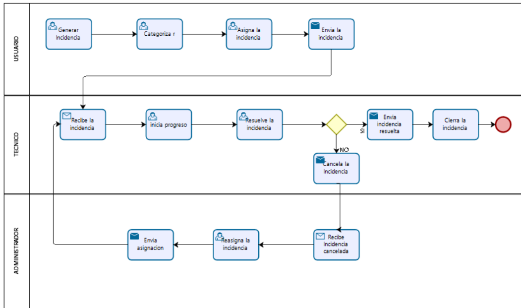
Figura. 3.2. Diagrama de procesos automatizado
