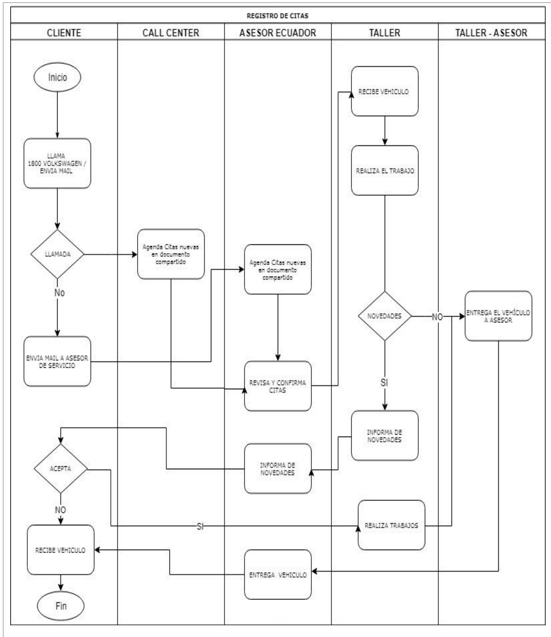
Figura 3.1. Diagrama de proceso actual
