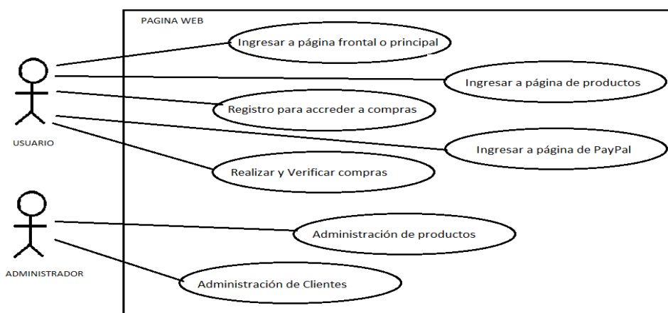
Figura 7: Diagrama de Casos de Uso
