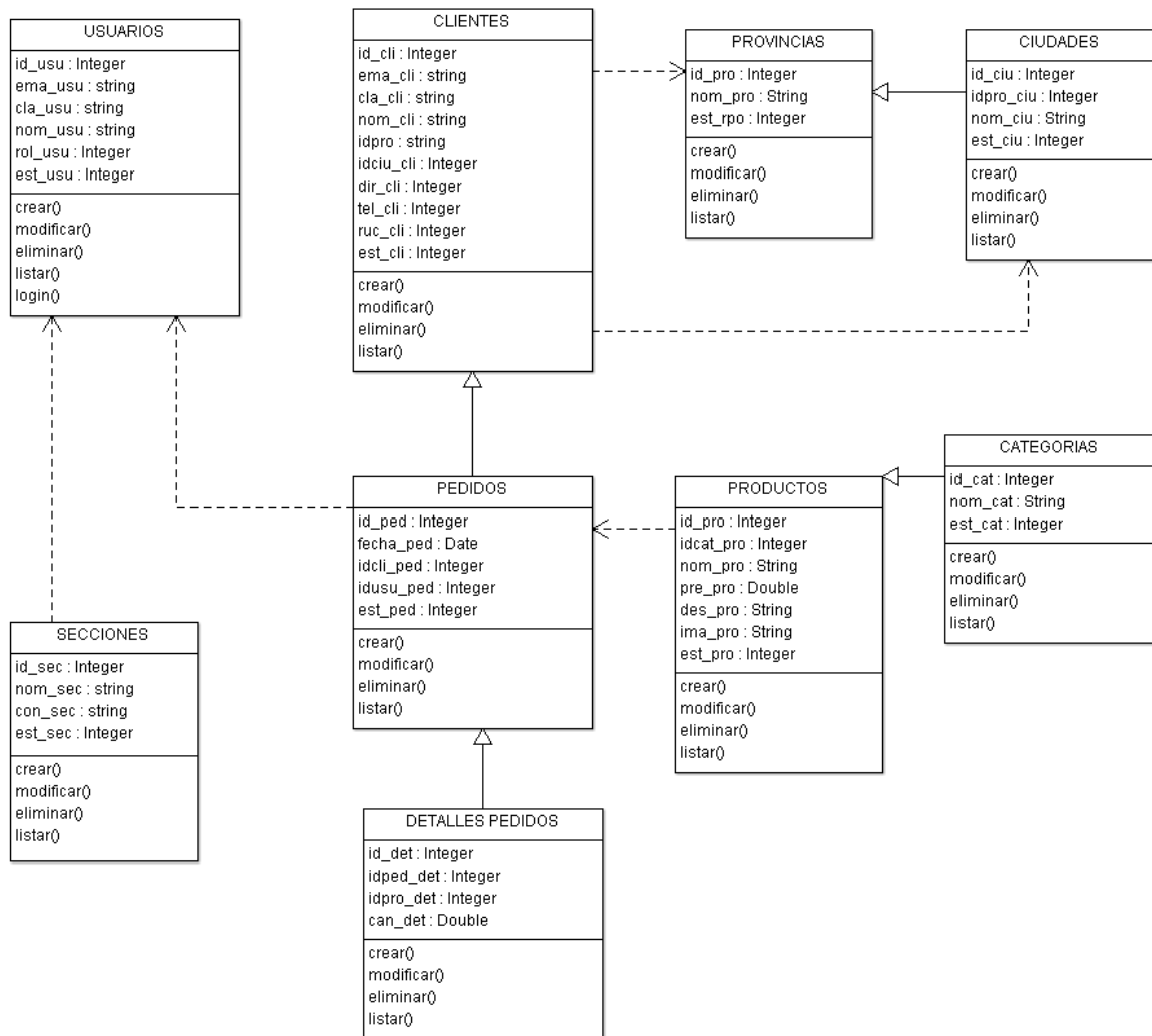
Figura 11: Diagrama de Clases
